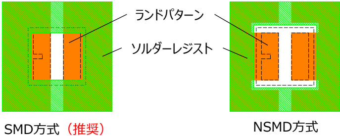
図10. ランドパターンの形成方法
