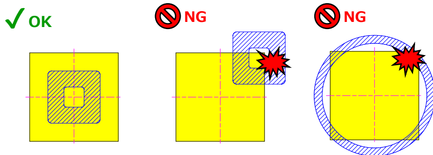
図14. 推奨吸着ノズル形状
