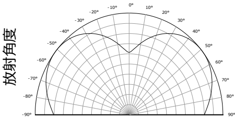
図8. 配光特性
