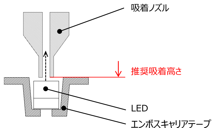
図16. 推奨吸着高さ
