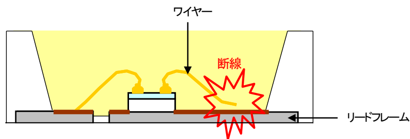
図 4. 不点灯メカニズム
