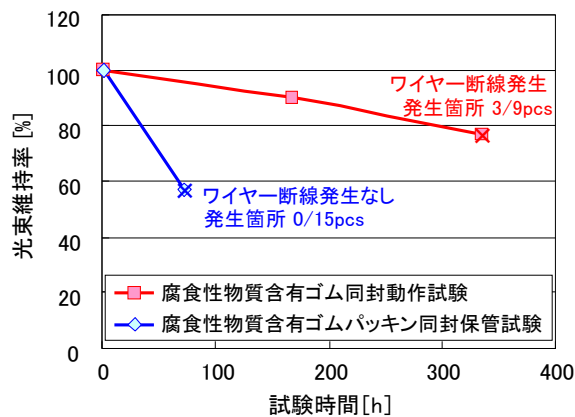
図 6. NS6W183A 硫化試験結果
