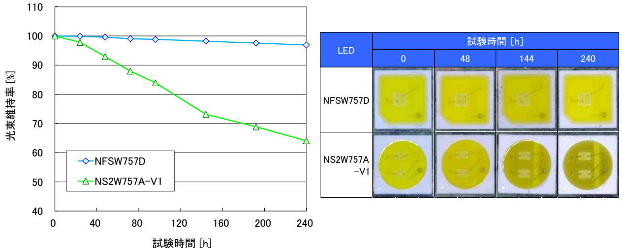
図 7. LED の硫化試験結果
