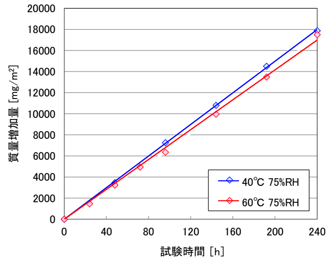
図 11. 銀板質量増加量
