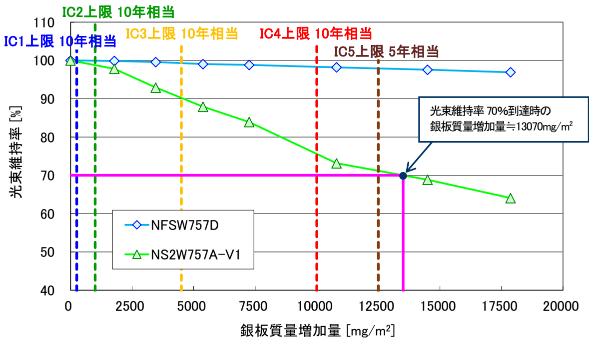
図9. 銀板質量増加量とLED 光束維持率
