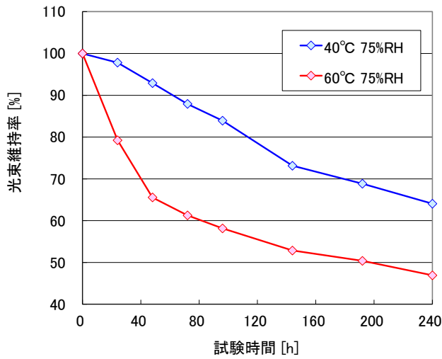
図 10. NS2W757A-V1 光束維持率
