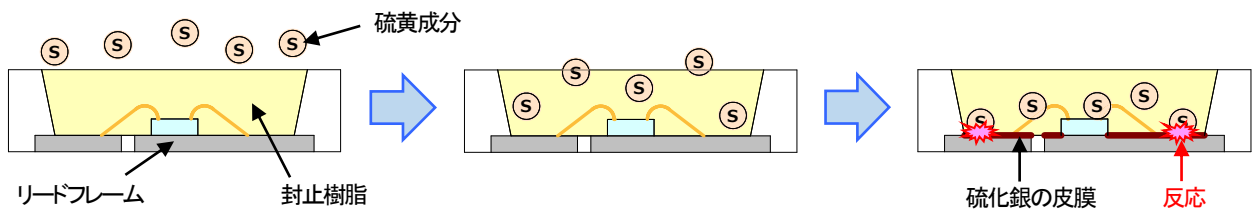
図 1. リードフレームの硫化概略図
