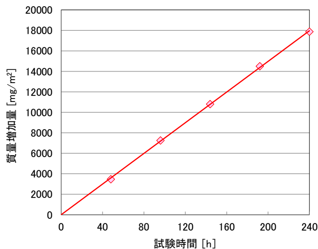
図 8. 腐食による銀板の質量増加量調査結果
