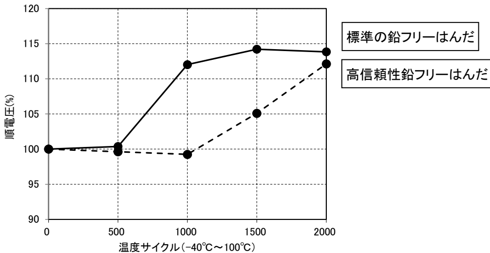
図 12. 温度サイクル試験結果(平均順電圧)
