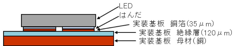
図3 実装構造
