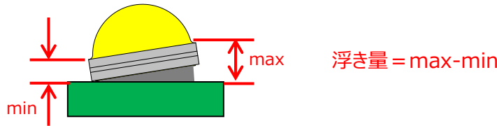
図12. 片浮き測定方法
