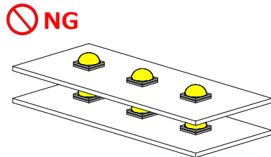
図2. 実装基板の不適切な取扱い例
