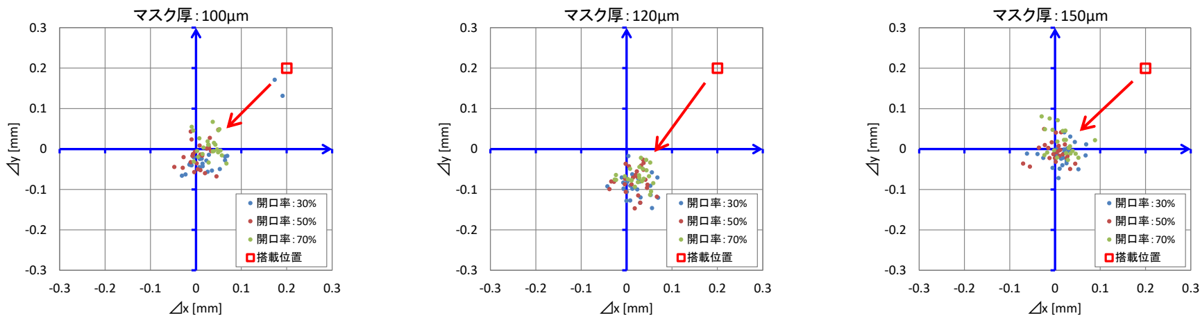
図13. 評価結果 (① x:+0.2mm,y:+0.2mm) ※n=各24pcs
