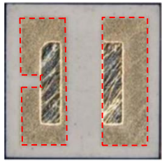
図3. 製品端子面外観
