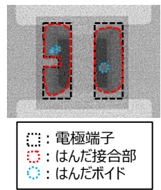
図5. 参考X線写真
