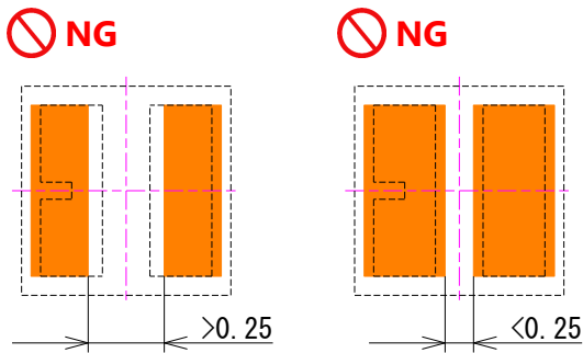
図2. 非推奨ランドパターン例
